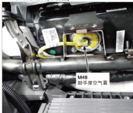
113.仪表板右侧(下视图)
