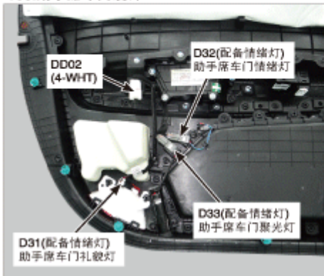
109.助手席车门装饰
