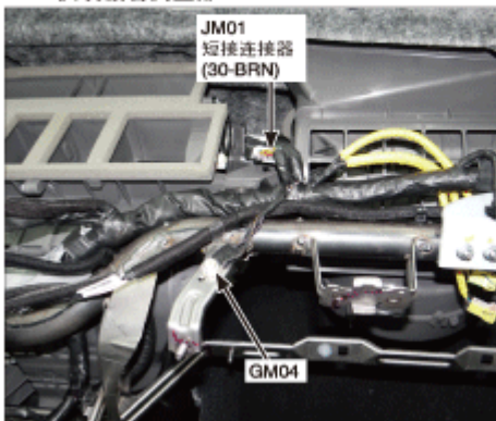
112.仪表板右侧上部
